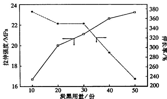
图1 炭黑用量对共混物拉伸强度和伸长率的影响
