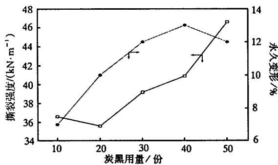
图2 炭黑用量对共混物撕裂强度和永久变形的影响
