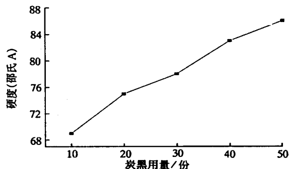
图4 炭黑用量对共混物硬度的影响
